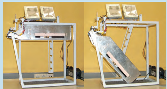
Abb. 6: Neigungsoptometer in Null und 50 Grad Position.
