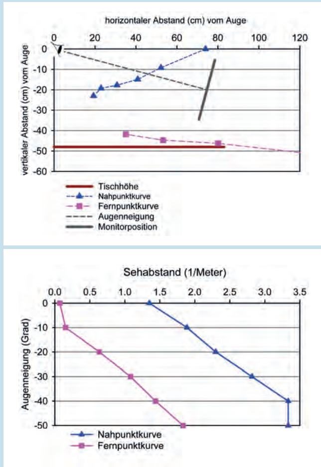
Abb. 8: Beispiel eines Ergebnis-Diagramms einer Schärfenbereichsmessung mit dem Neigungsoptometer. (Obere Abbildung: Arbeitsplatzdarstellung; untere Abbildung: optometrische Darstellung).
